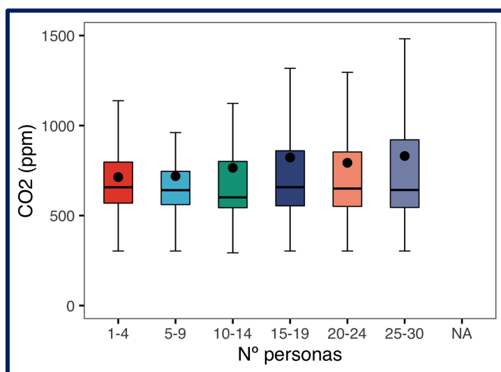
Gráfica 66: Boxplot con valores medios de CO 2 en función del número de personas
