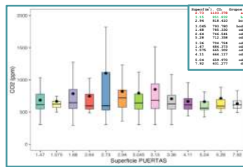
GRÁFICA 5: VALORES MEDIOS DE CO 2 EN FUNCIÓN DE LA SUPERFICIE DE ENTRADA Y SALIDA DE AIRE POR LAS PUERTAS
