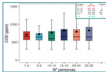
GRÁFICA 4: VALORES MEDIOS DE CO 2 EN FUNCIÓN DEL NÚMERO DE PERSONAS
