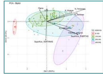
GRÁFICA 10: GRÁFICO BIPLLOT REPRESENTANDO AGRUPAMIENTO POR VOLUMEN DE LA ESTANCIA.
